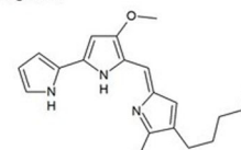
Prodigiosin
